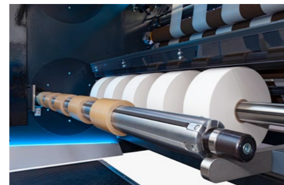
气胀轴 用于简单的应用。
