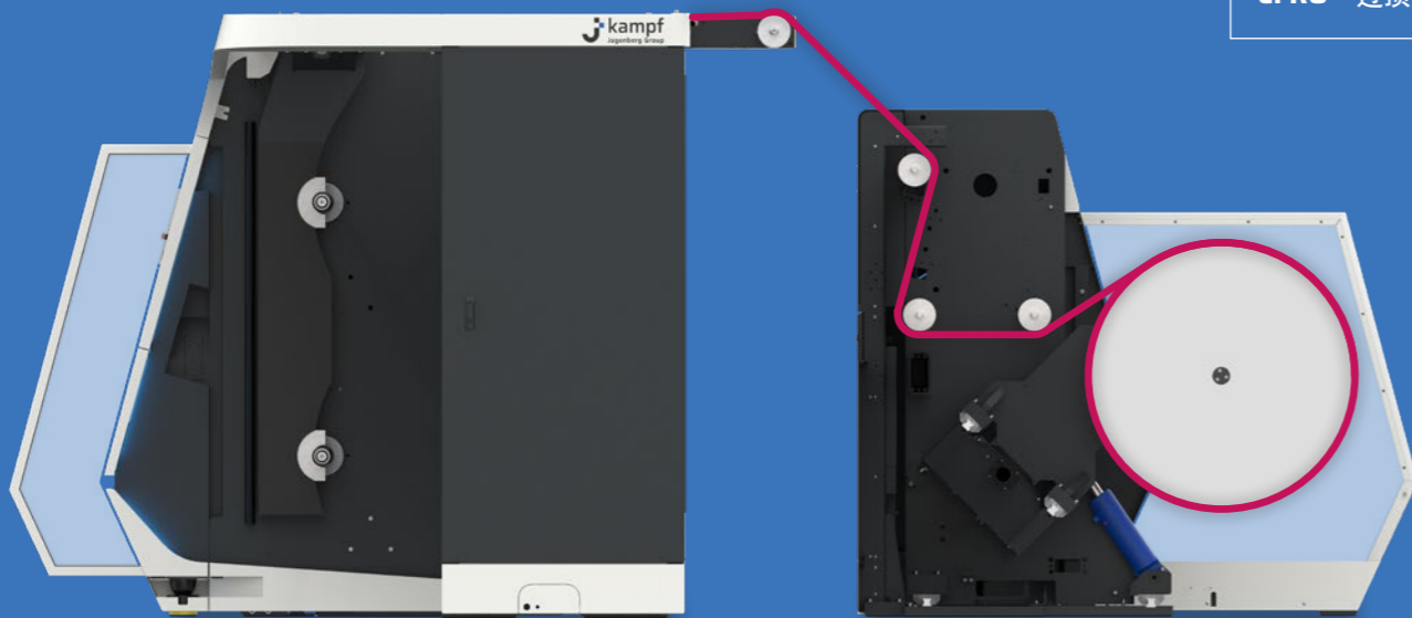
CFRO - 过顶穿料
