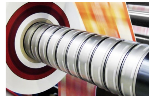
气涨和滑擦收卷轴 用于大批量的简单材料的生产或高要求材料的稳定质量生产。
